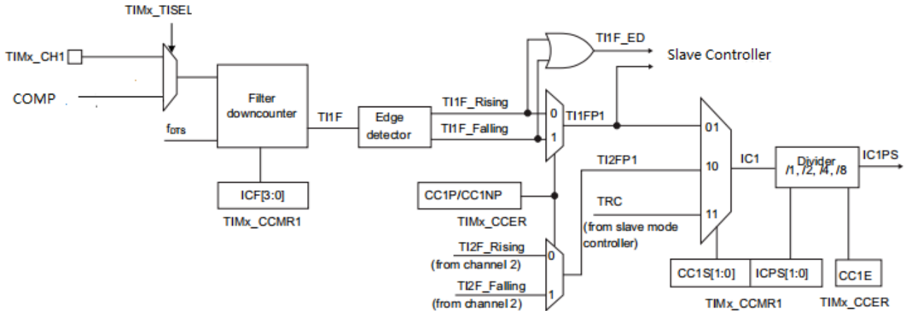
图 8-7 通道 1 输入捕获 TI1 信号
