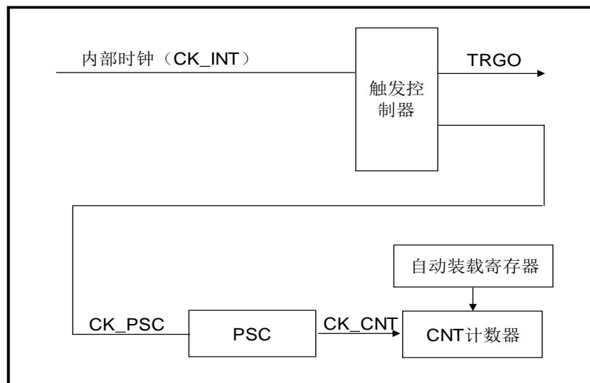
图 10-1 基本定时器 TIM6 结构框图
