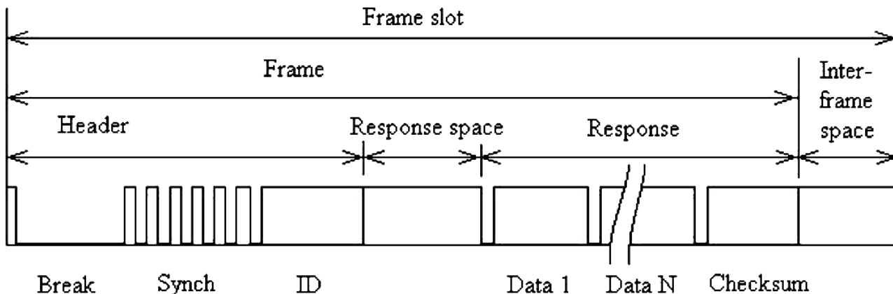
图 19-4 LIN 帧格式
