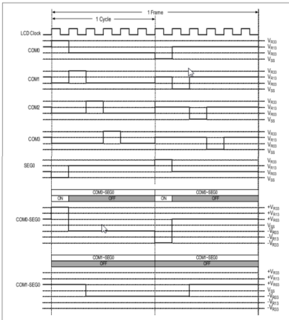
图 27-3 1/6 占空比 1/3 偏压 B 类波形图
