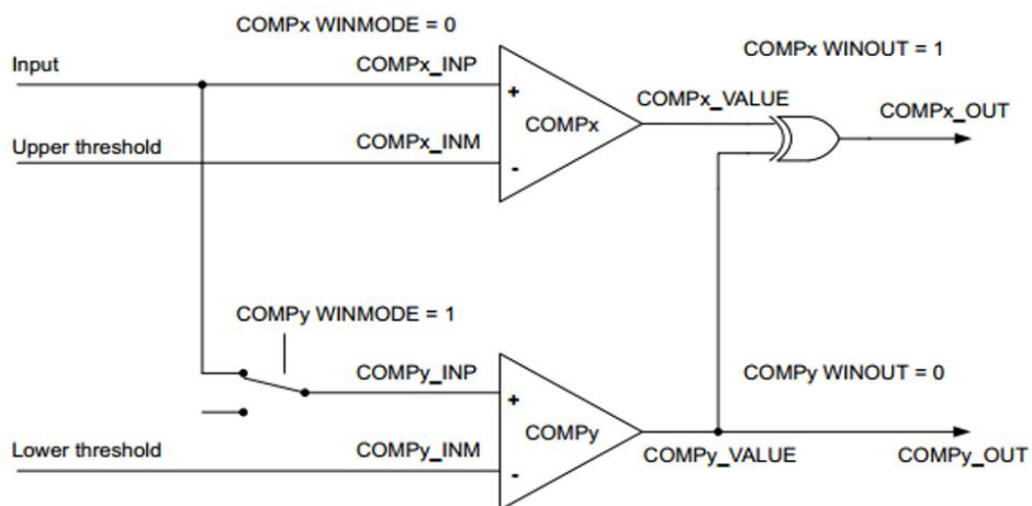
图 24-2 比较器窗口模式级联
