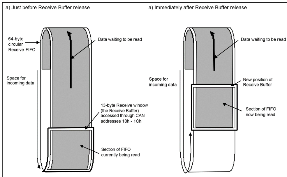
图 26-8 CAN 接收示意图
