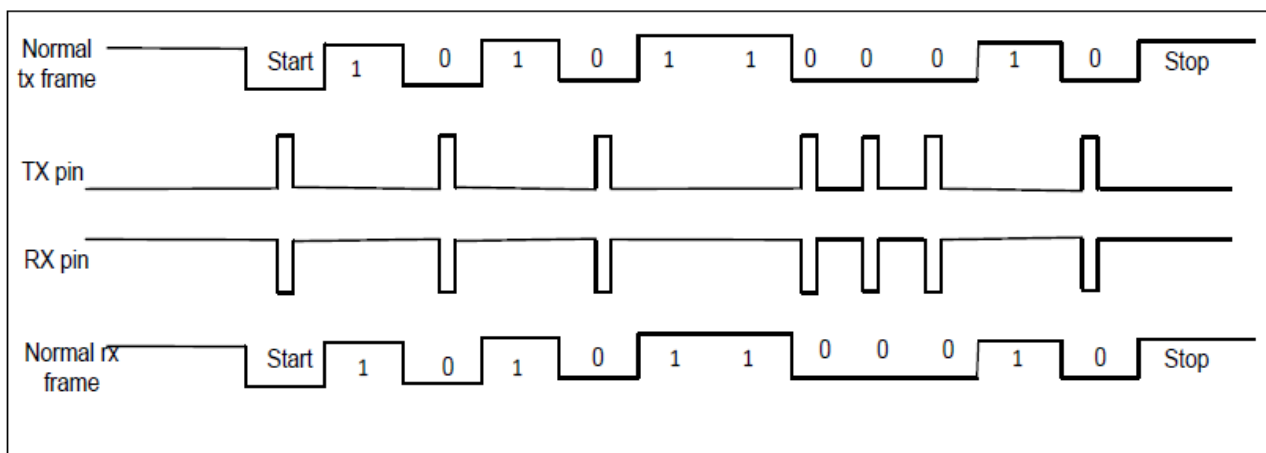
图 19-7 IrDA SIR 数据调制解调
