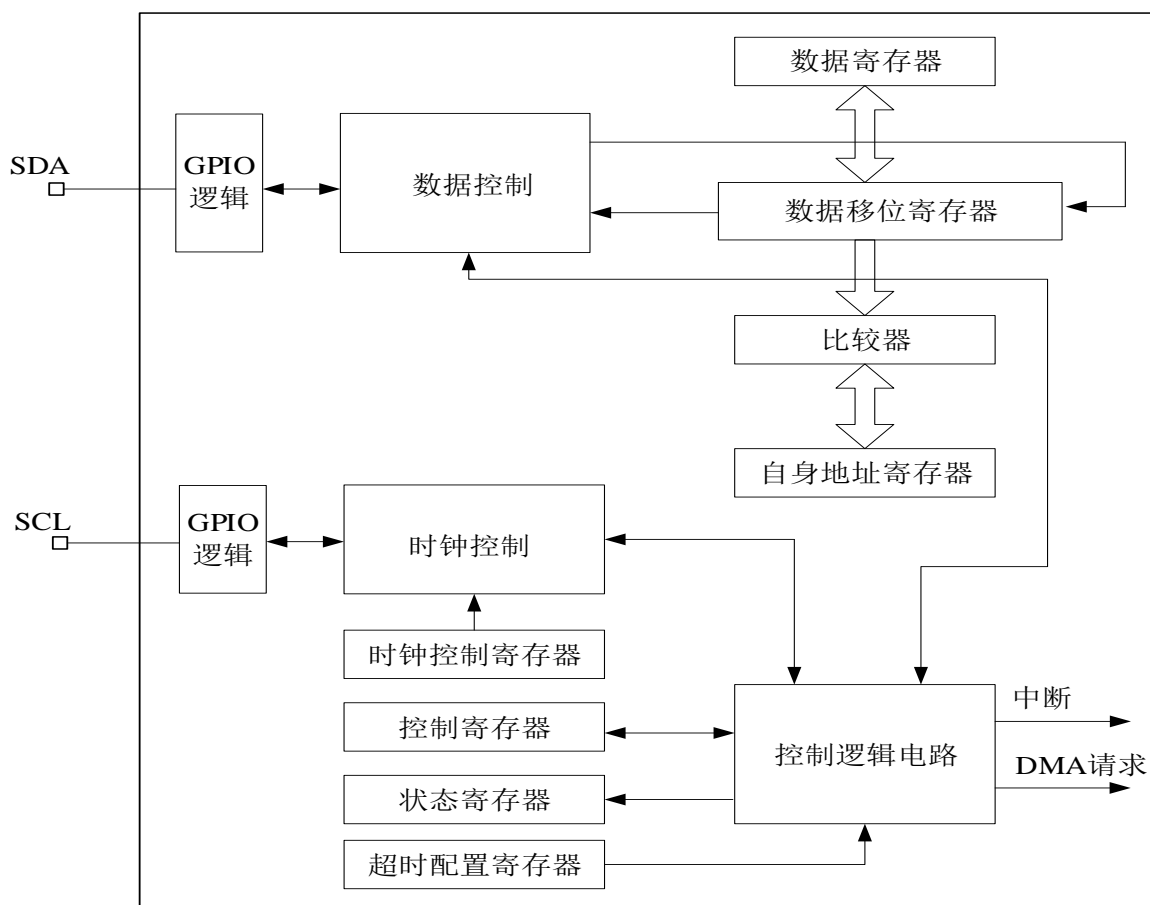
图 20-1 I2C 结构框图
