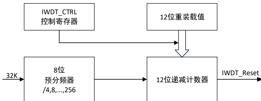
图 14-1 IWDT 框图
