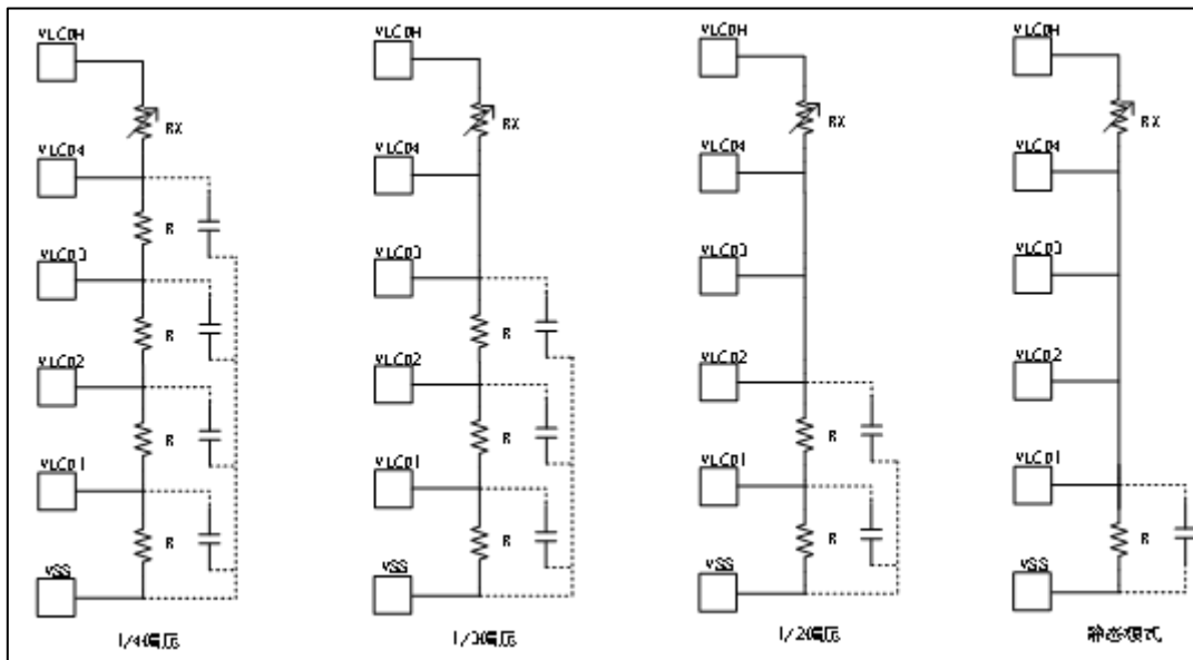
图 27-6 外部电阻模式连接示意图
