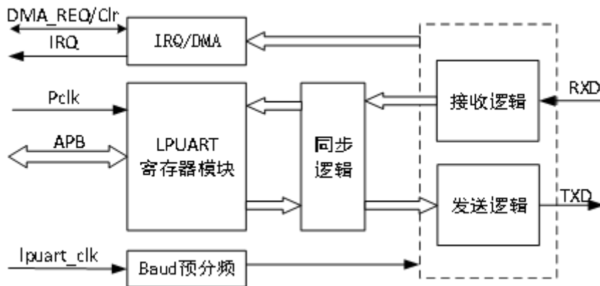
图 21-1 LPUART 整体框图
