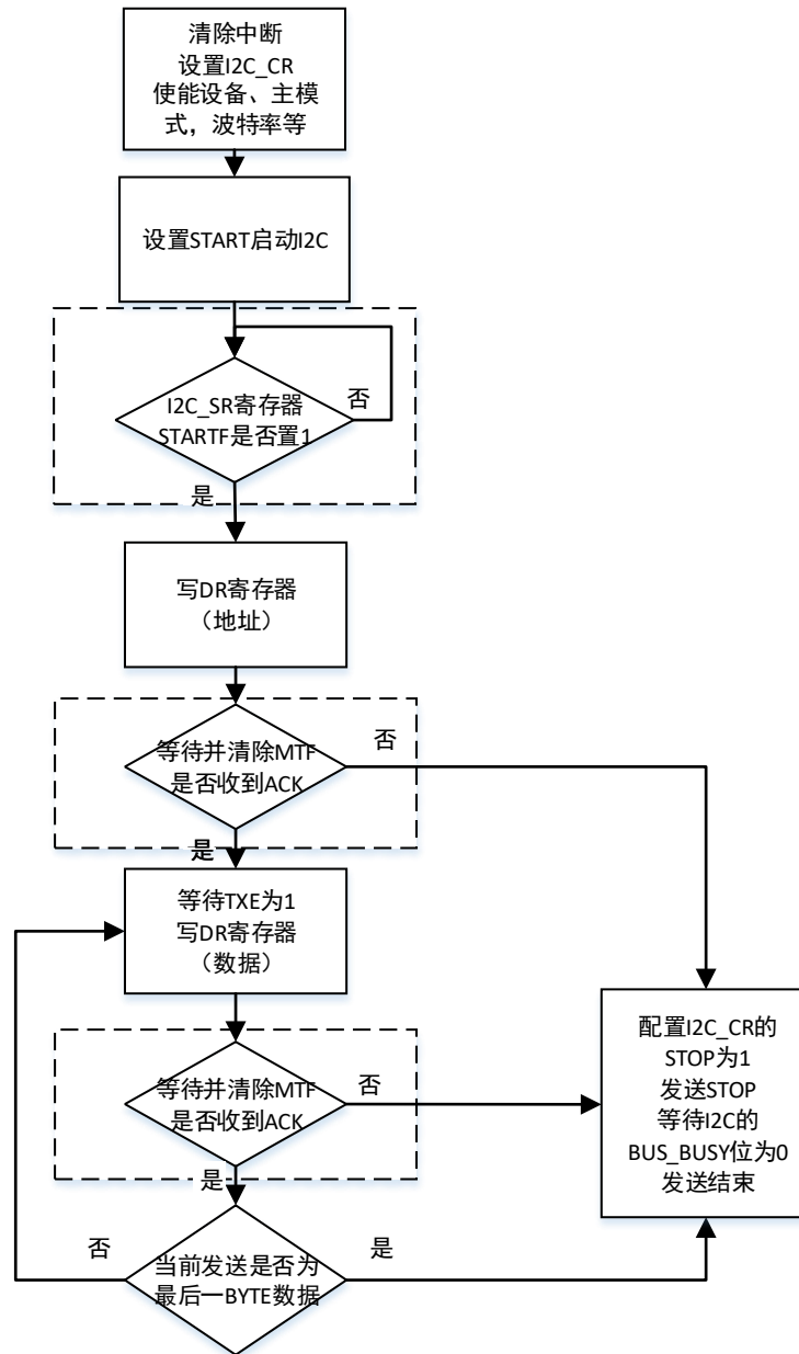
图 20-9 主机发送流程图 (虚线步骤可跳过, 下同)
