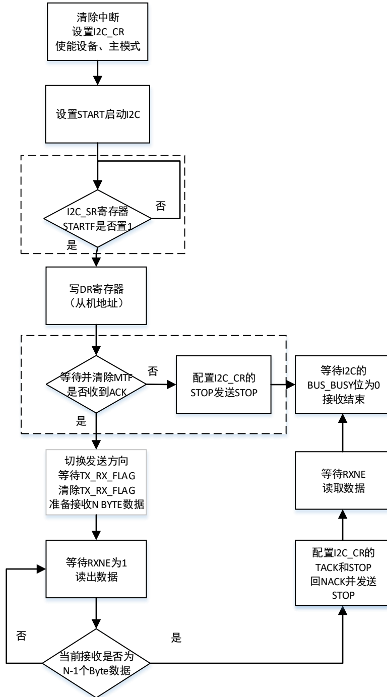
图 20-10 主机接收流程图
