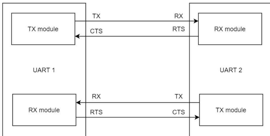
图 19-2 两个 UART 之间的硬件流控连接示意图
