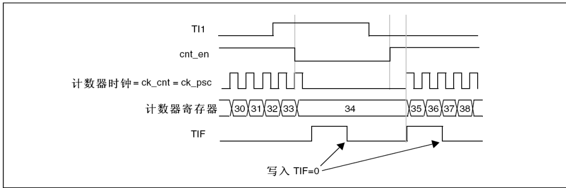
图 8-22 门控模式下的控制电路
