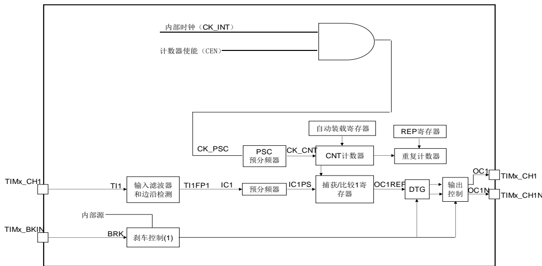
图 12-2 通用定时器 TIM16/TIM17 结构框图
