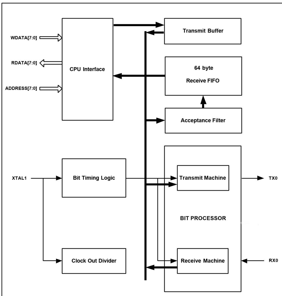
图 26-1 内部功能框图
