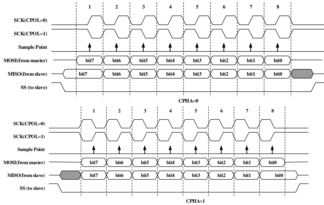
图 18-2 SPI 一线模式时序图 (MSB)
