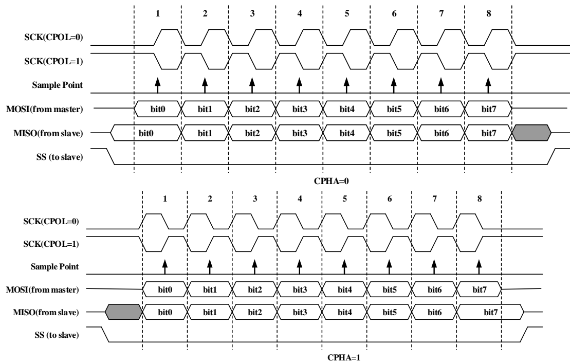
图 18-3 SPI 一线模式时序图 (LSB)
