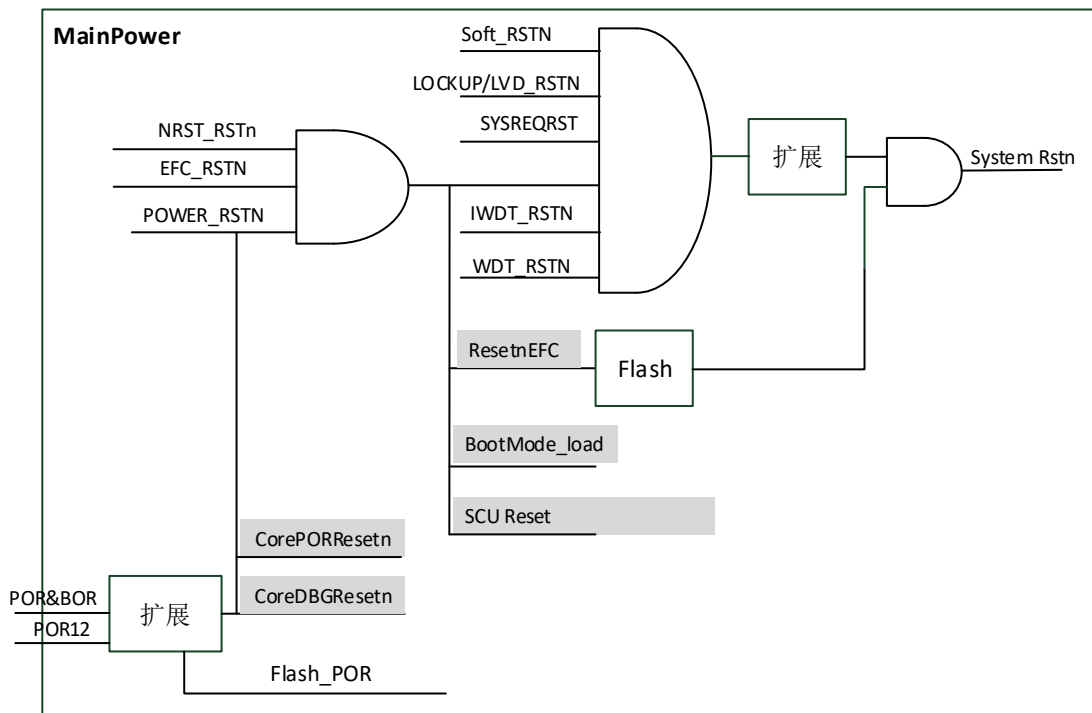
图 3-1 复位关系图
