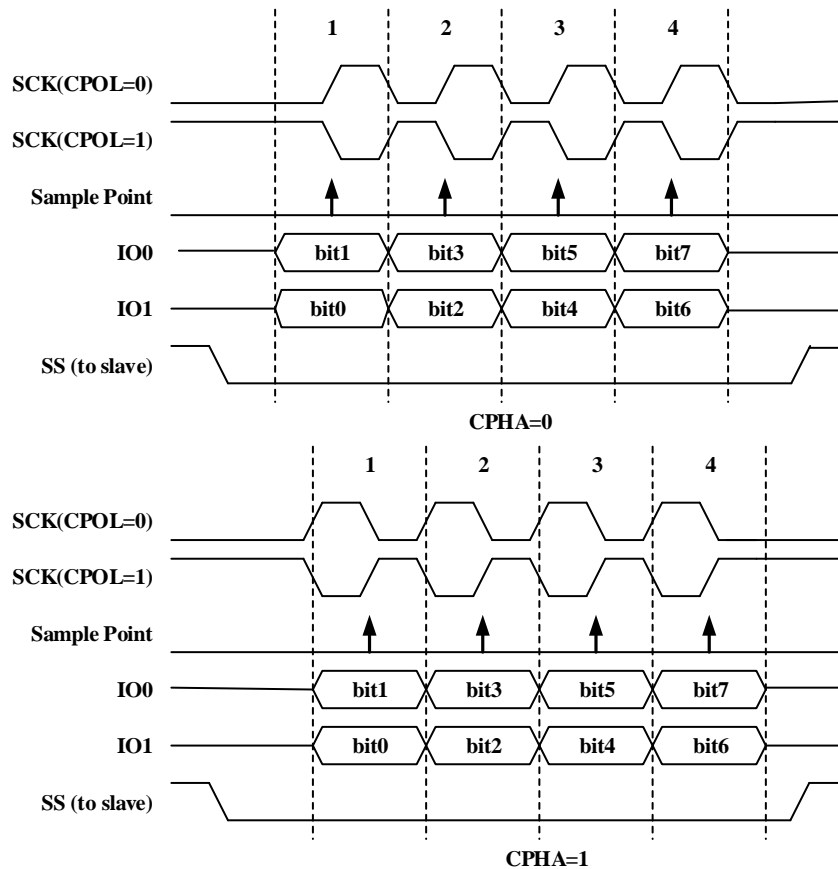
图 18-5 SPI 二线模式时序图 (LSB)
