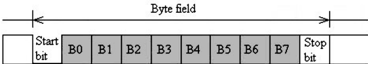
图 19-6 LIN 字符格式
