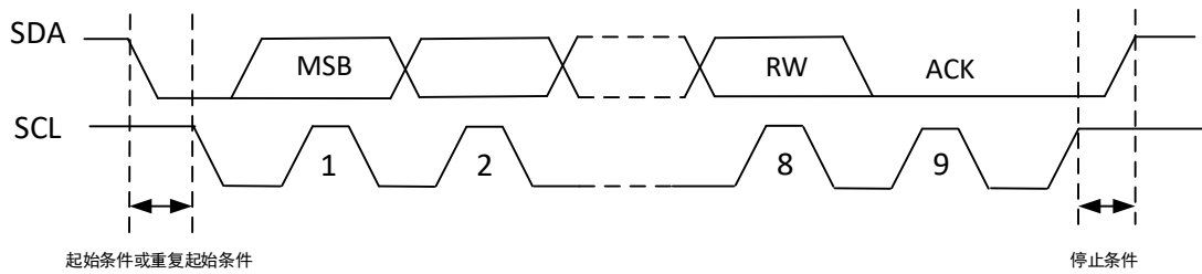
图 20-2 I2C 总线传输
