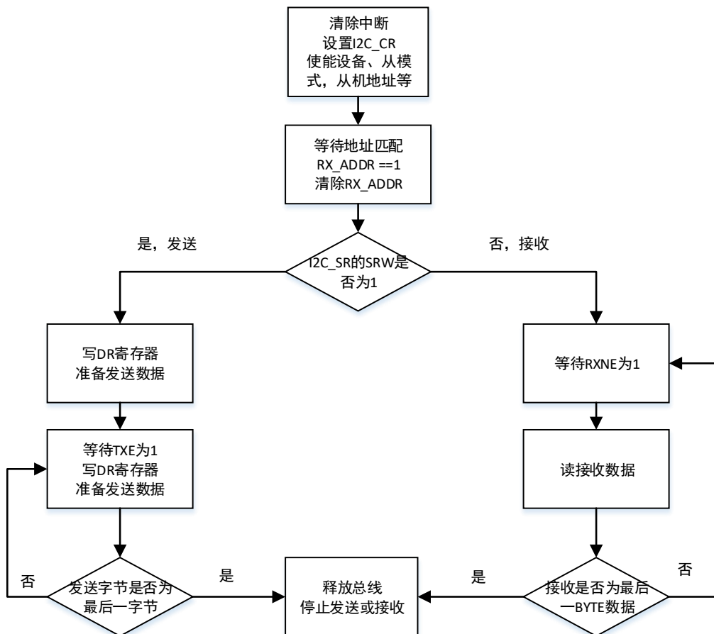
图 20-11 从机发送接收流程图
