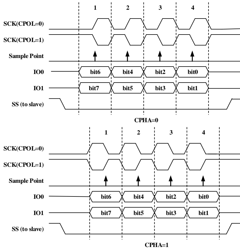
图 18-4 SPI 二线模式时序图 (MSB)
