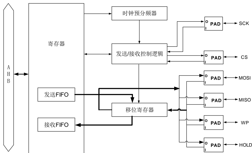
图 18-1 SPI 结构框图
