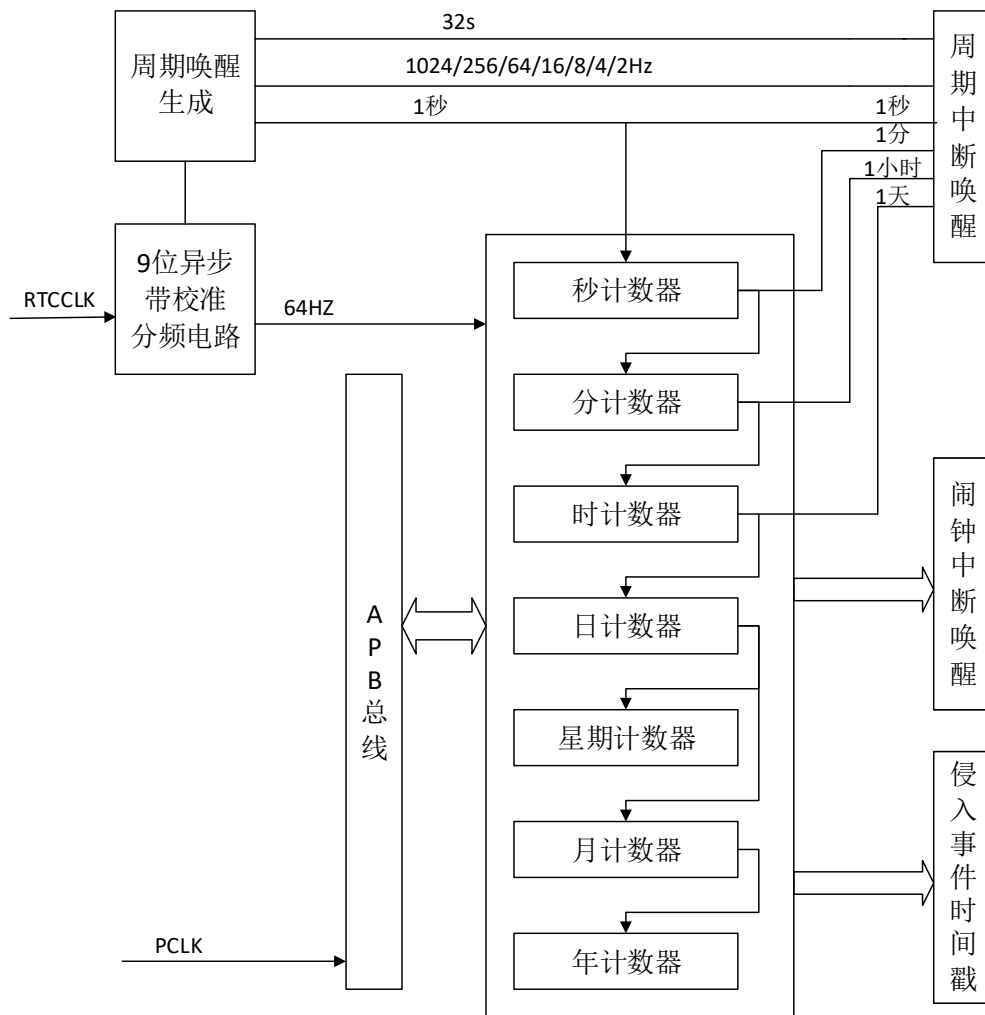
图 15-1 RTC 内部结构框图
