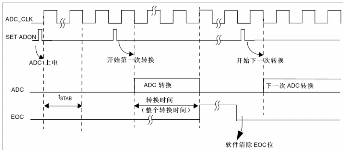
图 22-2 ADC 转换时序图
