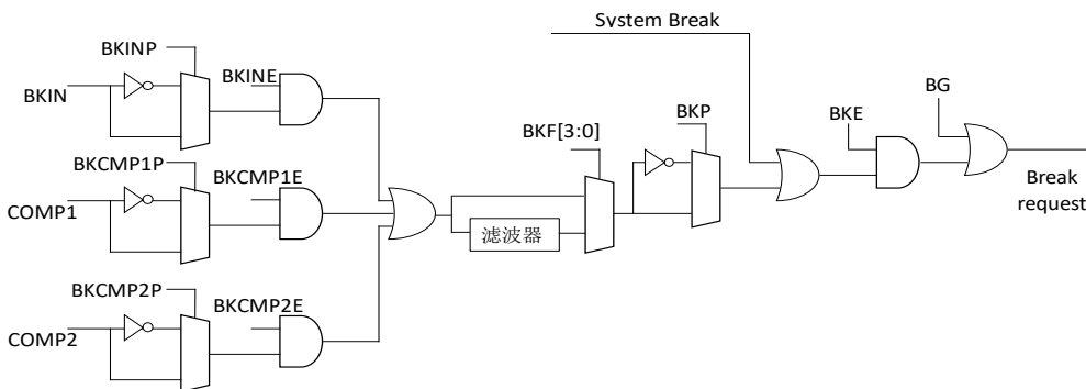
图 8-16 刹车控制
