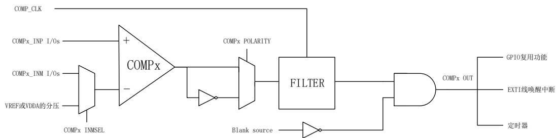
图 24-1 COMP 结构框图
