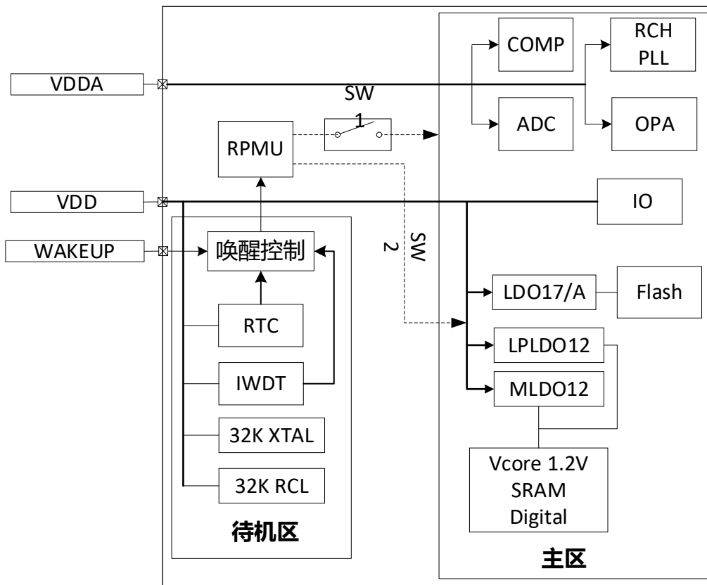
图 2-5 芯片电源域
