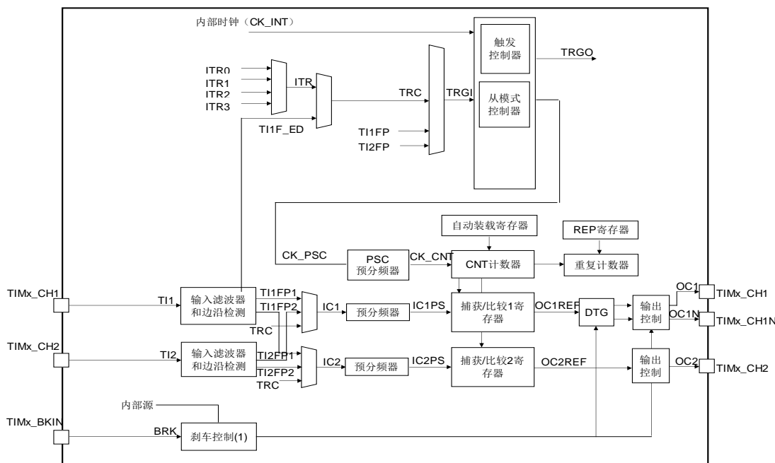
图 12-1 通用定时器 TIM15 结构框图
