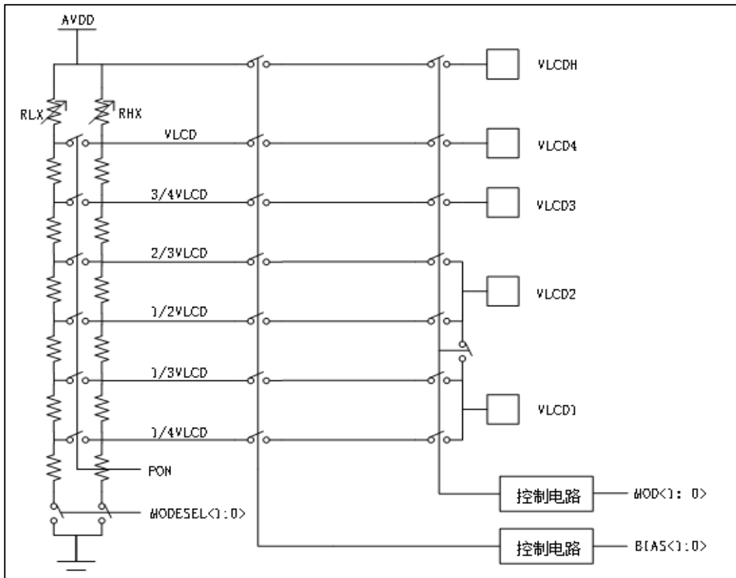
图 27-4 内部电阻分压电路示意图
