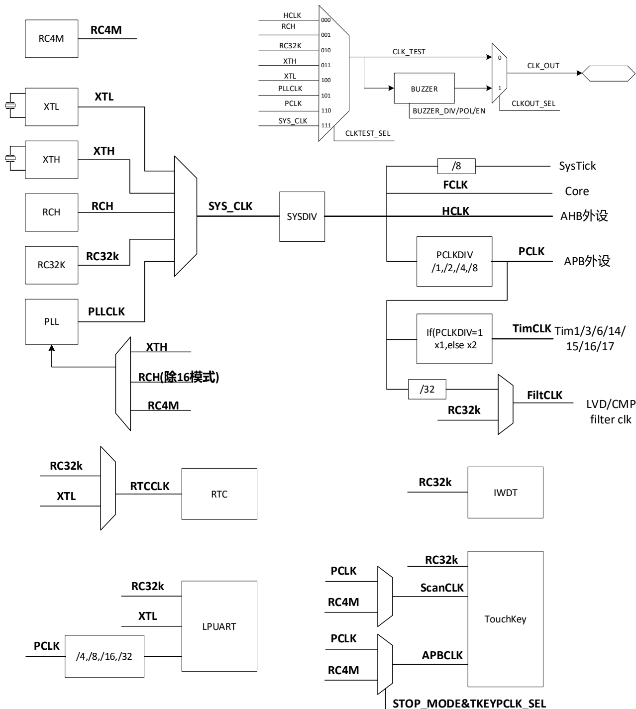
图 3-2 时钟结构图
