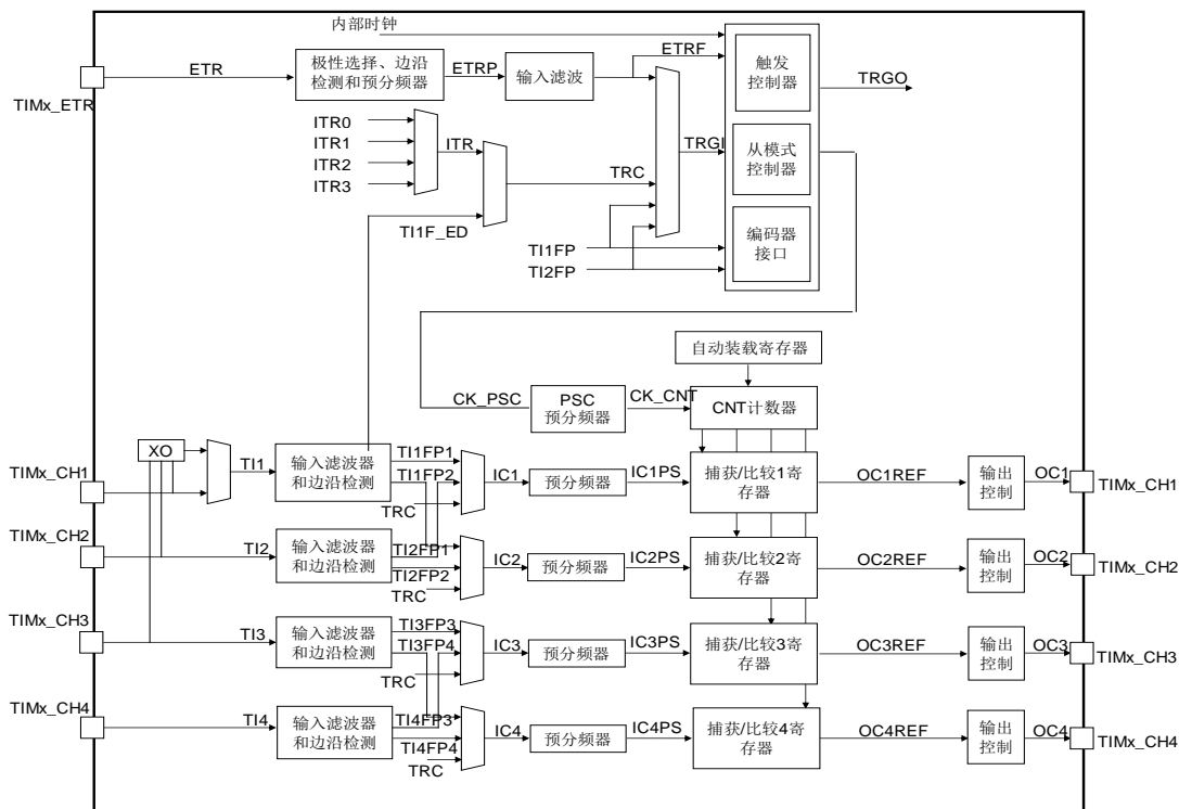
图 9-1 通用定时器 TIM3 框图
