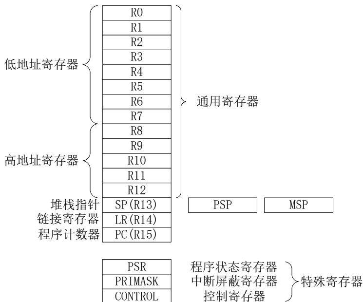
图 2-2 处理器寄存器组
