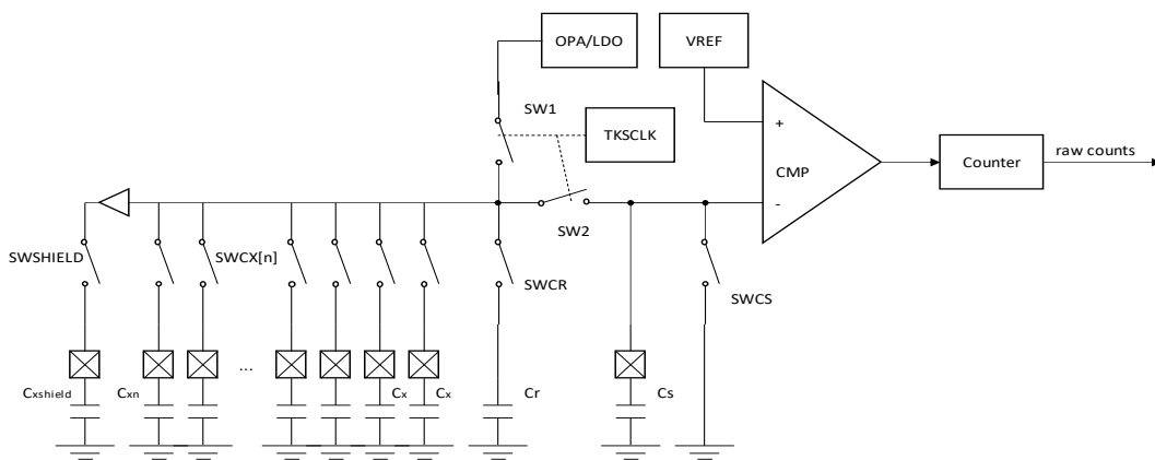
图 25-1 TKEY 结构框图
