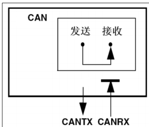
图 26-4 自测试模式示意图
