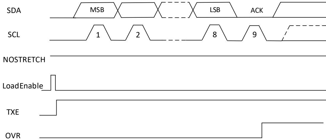
图 20-5 从机发送模式时钟延长时序 (虚线部分 SCL 为低, 主机无法发送 SCL)
