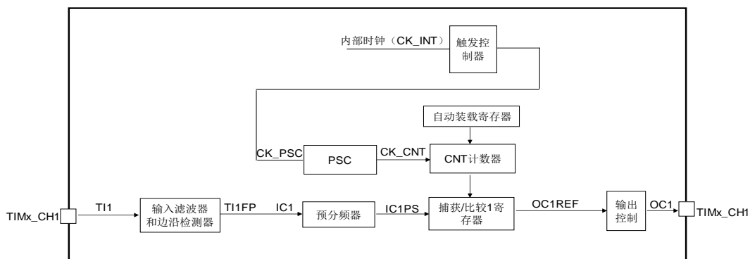
图 11-1 通用定时器 TIM14 结构框图
