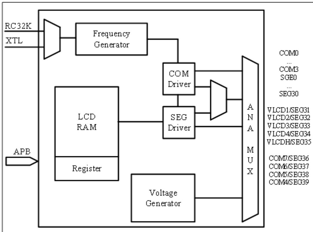
图 27-1 LCD 系统框图
