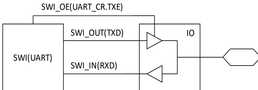
图 19-8 UART 单线半双工模式框图
