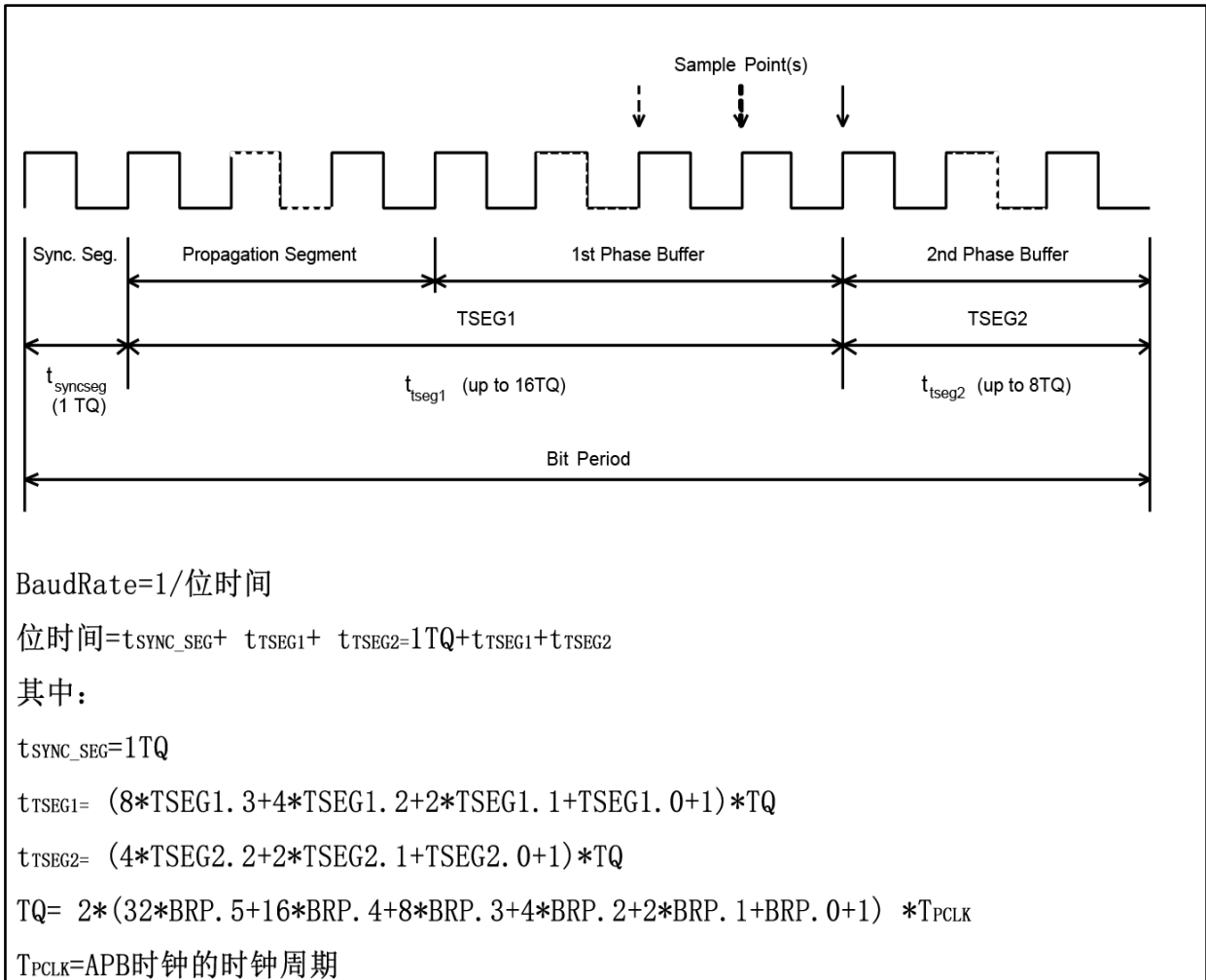
图 26-11 CAN 位时序图
