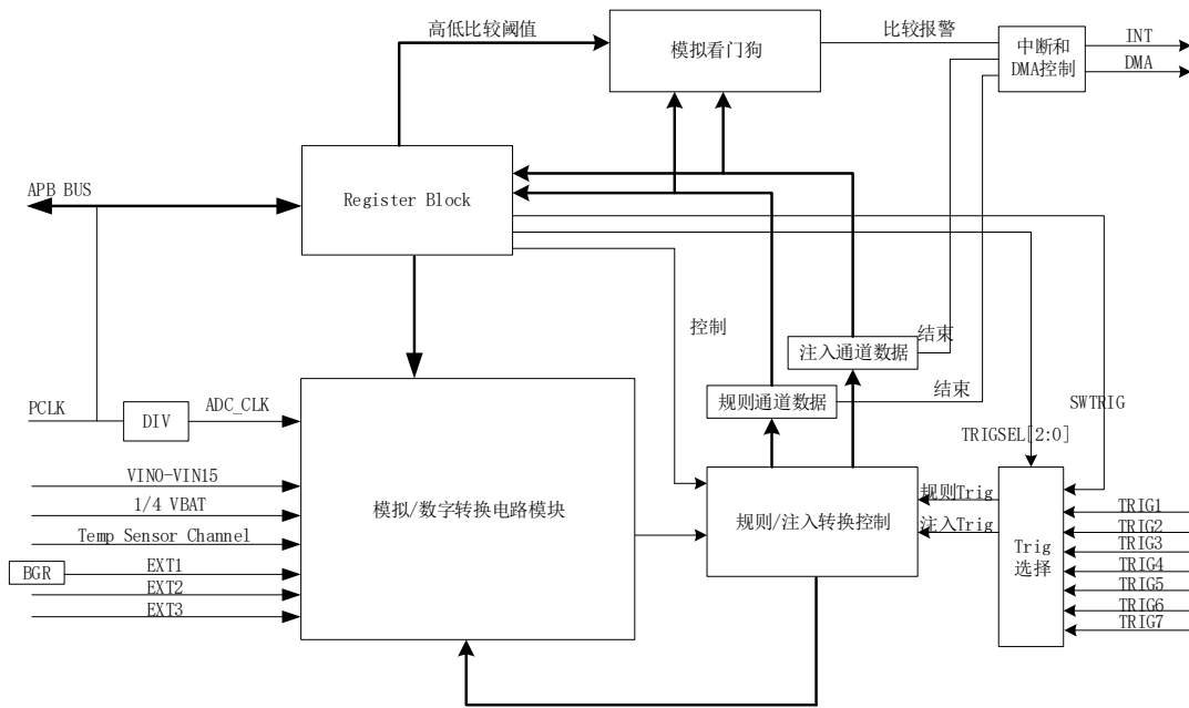
图 22-1 ADC 框图
