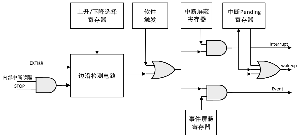
图 5-1 EXTI 系统框图
