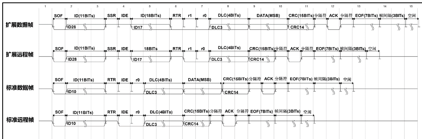
图 26-5 CAN 数据帧结构
