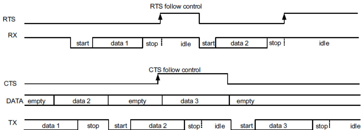
图 19-3 硬件流控时序图
