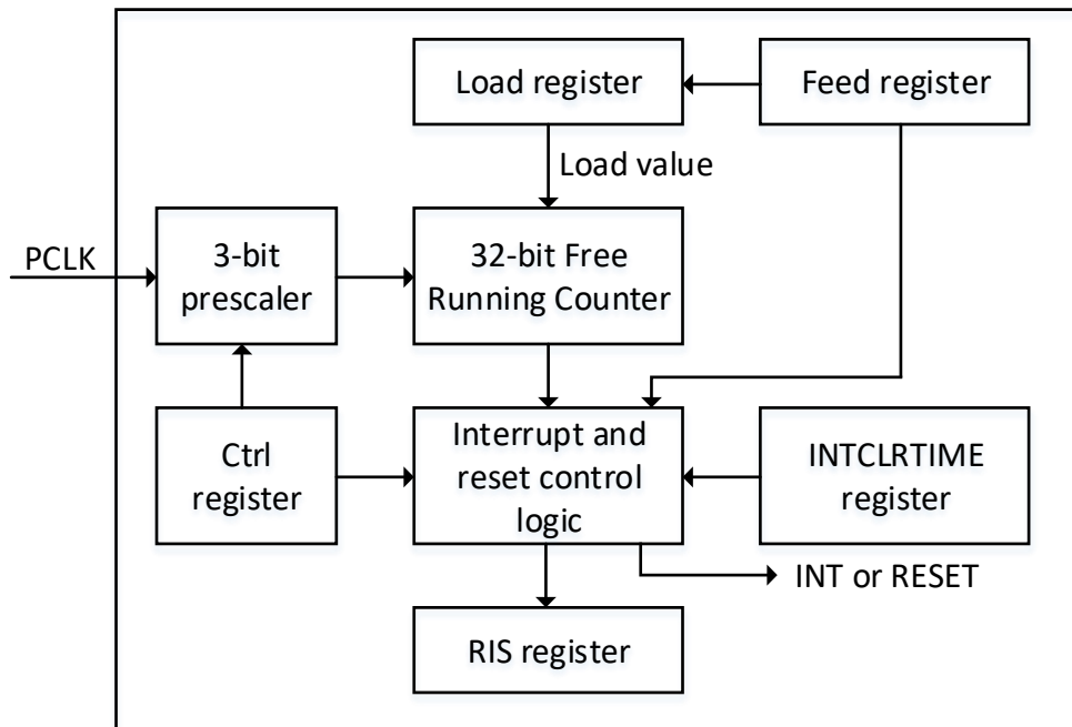
图 13-1 WDT 功能框图
