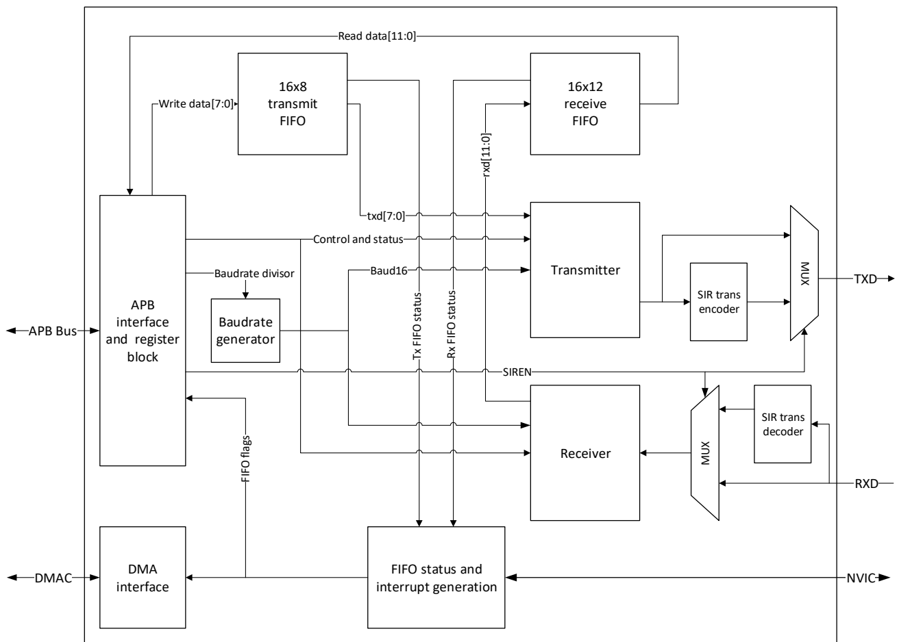
图 19-1 UART 结构框图
