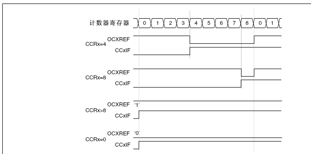
图 8-10 边沿对齐的 PWM 波形 (ARR=8)
