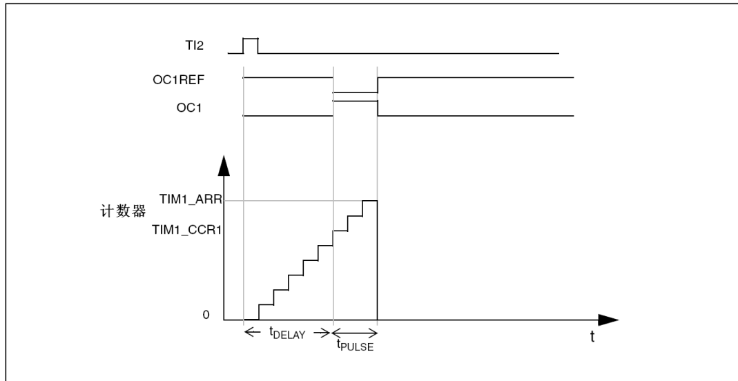
图 8-20 单脉冲模式的例子
