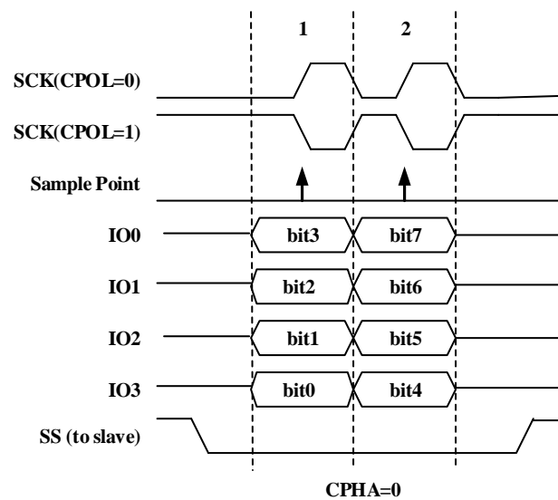
图 18-7 SPI 四线模式时序图 (LSB)
