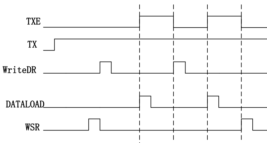
图 20-8 TXE 功能说明图
