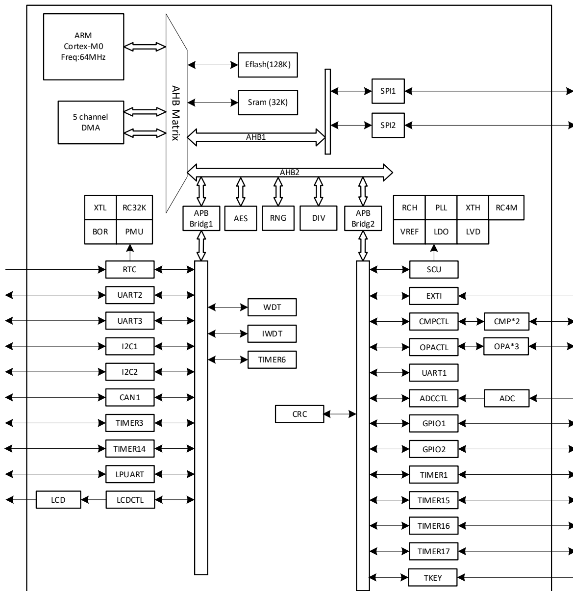
图 2-3 芯片系统架构图
