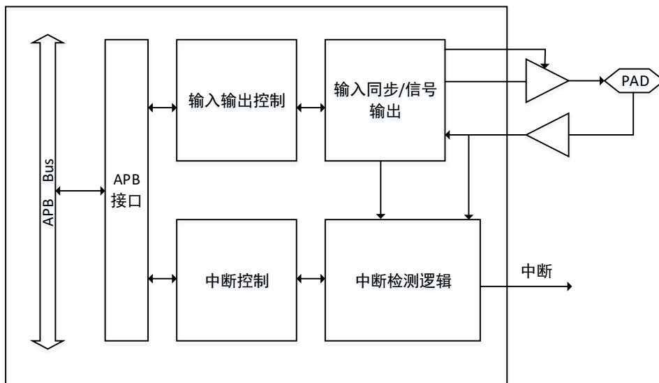
图 17-1 GPIO 结构框图
