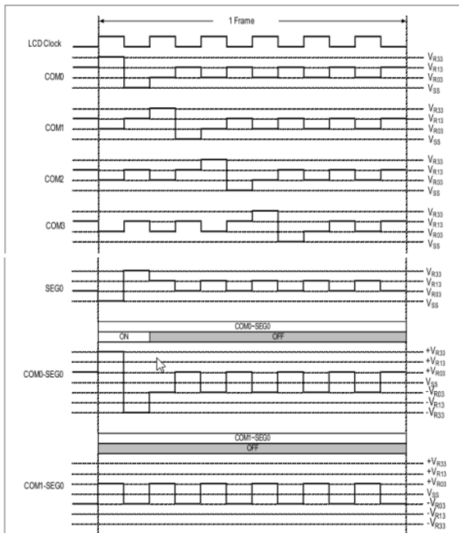
图 27-2 1/6 占空比 1/3 偏压 A 类波形图
