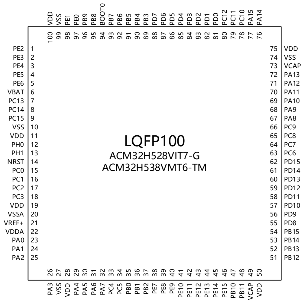
图 3-1 LQFP100 封装管脚分布图
